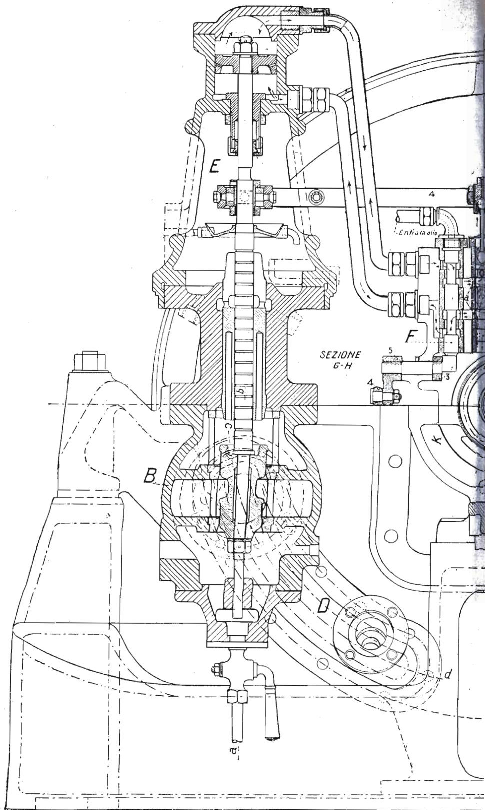
Fig. 330. — Sistemazione della distribuzi
