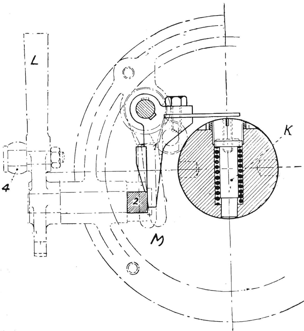
Fig. 331. Sezione e-f
