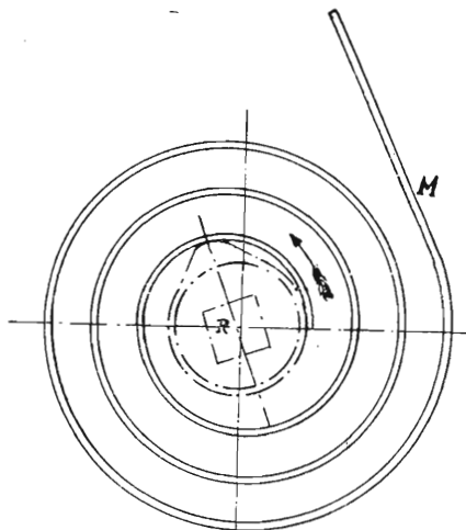
Fig. 317 Azione della molla del nottolino secondo la freccia
