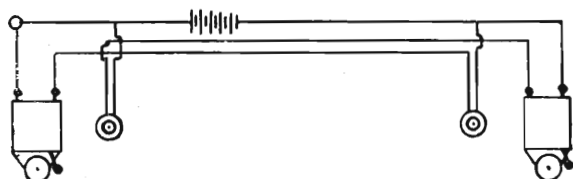
Impianto di due suonerie coa c'hamata reciproca
