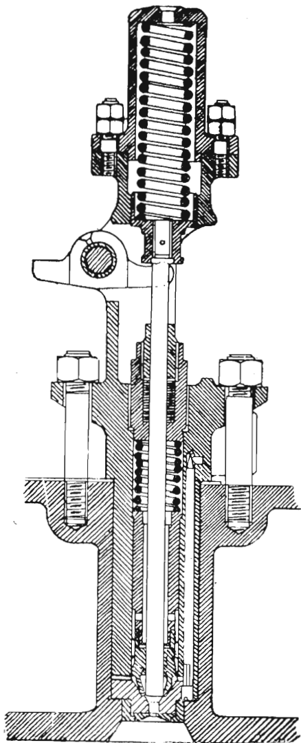
Fig. 349. Polverizzatore
