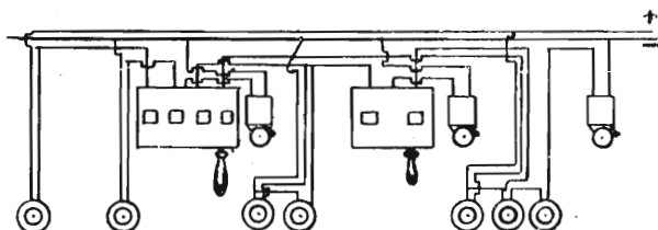
Impianto multiplo con quadri indicatori
