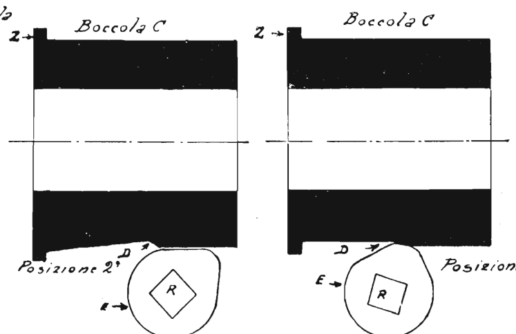
Posizione del nottolino al momento dello scatto (così la valvola è chiusa)
